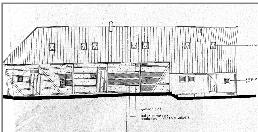
Bouwtekening achtergevel
