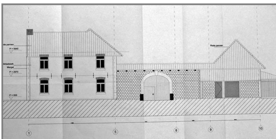
Bouwtekening van de voorgevel
